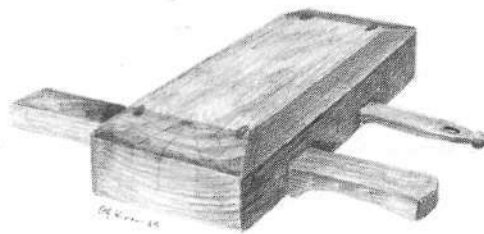
Puukoneistoinen puulukko, haapaa. Pielisjärvi. KM. B 123. Tavallisesti koppa tehtiin koivusta.
