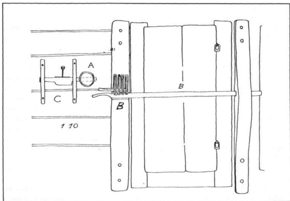
Nivelavaimella avataan salpa ja aukon A kautta käsi työnnetään avaimineen sisään ja avataan puulukko B.
