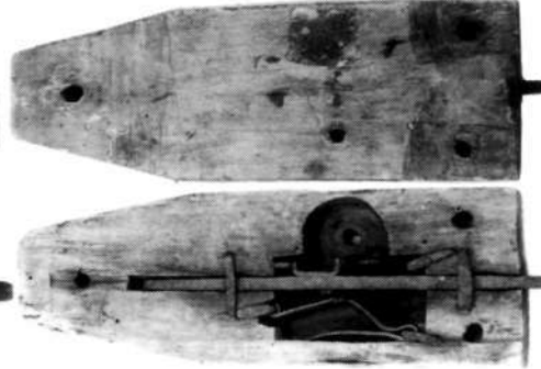
Eestiläinen vaakasuora puukoppalukko. Tehty 1860, Ambla, Tarton kansatiet. museo.
