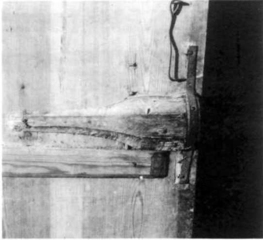
Aitan vaakasuora lukko. Valok. Alfred Kolehmainen. Murtovaara, Valtimo.
