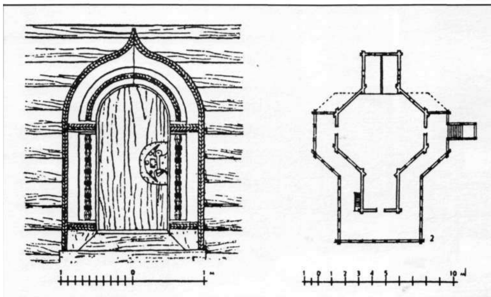
Portaali Ishne-joen varrella sijaitsevasta 1687 vuoden kirkosta Bogoslovskin-kylässä. Piirros teoksesta: "Istoriija russkoi arhitektury", Moskva 1956.
