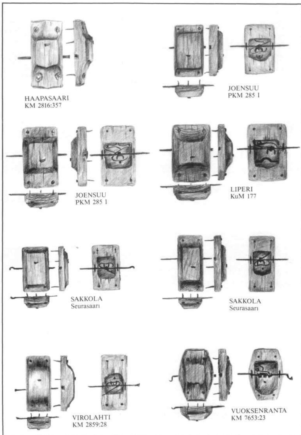
Karjalaisia rautakoneistoisia pystykoppalukkoja
