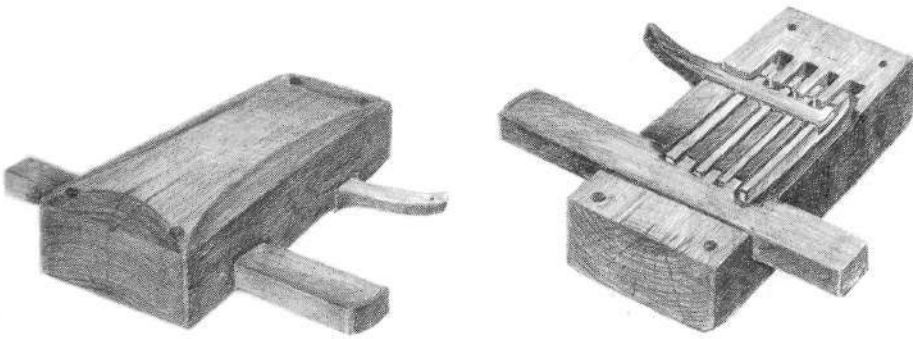
Rääkkylän puulukko päältä ja koneiston puolelta katsottuna.
