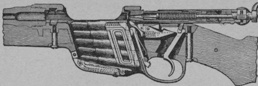
Kuva 4. Itävaltalaisen Mannlicher-kiväärin lukko-osa.
