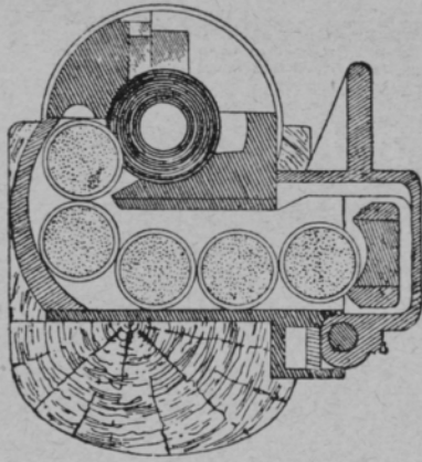
Ku va 7. Krag-Jörgensen-makasiini täytettynä.
