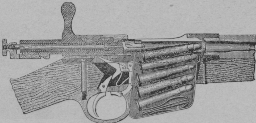
Kuva 3. Irroitettavalla Lee-makasiinilla varustetun kiväärin lukko-osa.
