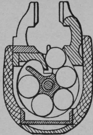
Ku va 8. Rumpumakasiinin poikkileikkaus.
