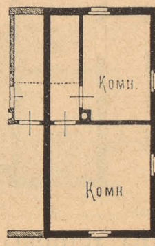
КАМЕННАЯ ДАЧА ДЛЯ ДВУХЪ СЕМЕЙСТВЪ ВЪ 9940 РУБ.
