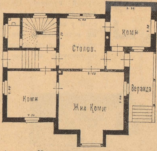
КАМЕННАЯ ДАЧА ДЛЯ ОДНОГО СЕМЕЙСТВА ВЪ 6800 РУБ.
