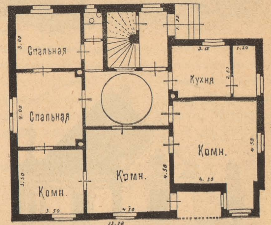
КАМЕННАЯ ДАЧА ДЛЯ ДВУХЪ СЕМЕЙСТВЪ ВЪ 9940 РУБ.
