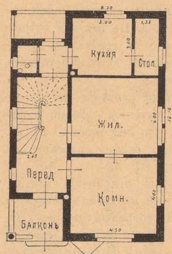
КАМЕННАЯ ДАЧА ДЛЯ ОДНОГО СЕМЕЙСТВА ВЪ 4950 РУБ.
