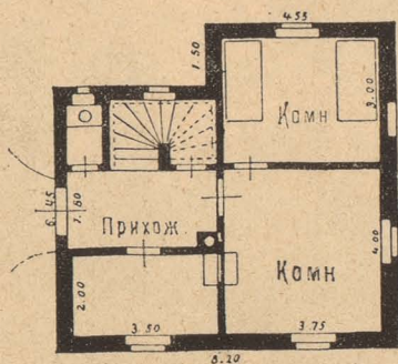
ДАЧА ДЛЯ ДВУХЪ НЕБОЛЬШИХЪ СЕМЕЙСТВЪ ВЪ 1800 РУБ.
