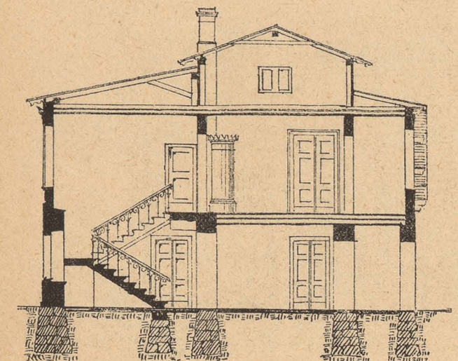
РАЗРѢЗЪ ДАЧИ ДЛЯ ОДНОГО СЕМЕЙСТВА
