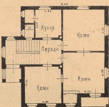
ЗАГОРОДНЫЙ ДОМЪ ДЛЯ ОДНОГО СЕМЕЙСТВА ВЪ 4550 РУБ.
