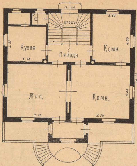
КАМЕННАЯ ДАЧА ВЪ 8000 РУБ.
