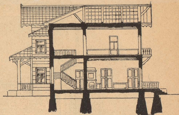
РАЗРѢЗЪ СЕЛЬСКАГО ДОМИКА
