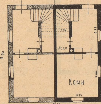
КАМЕННАЯ ДАЧА ДЛЯ ДВУХЪ СЕМЕЙСТВЪ ВЪ 990 РУБ.
