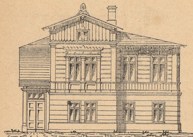
ПЕРЕДНІЙ ФАСАДЪ ДАЧИ ДЛЯ ОДНОГО СЕМЕЙСТВА
